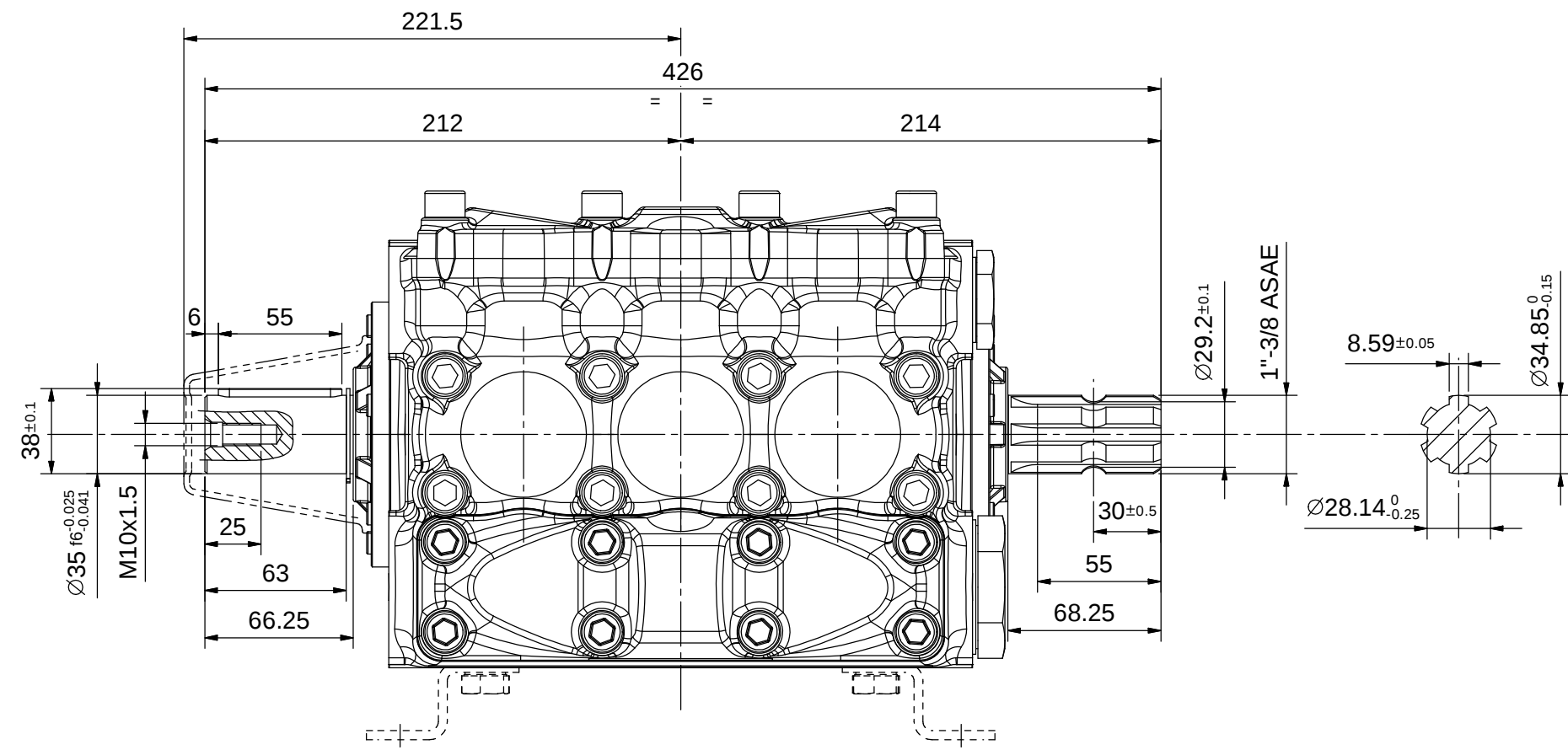
VERSIONE DOPPIA PRESA DI FORZA DIAM.35 - 1"-3/8 ASAE
