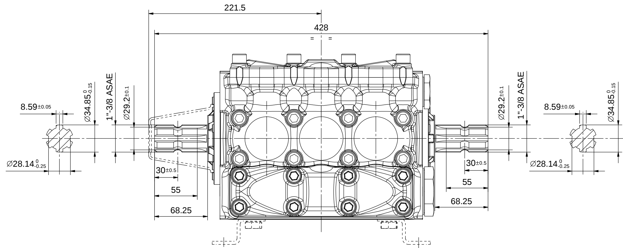
VERSIONE DOPPIA PRESA DI FORZA 1"-3/8 ASAE
