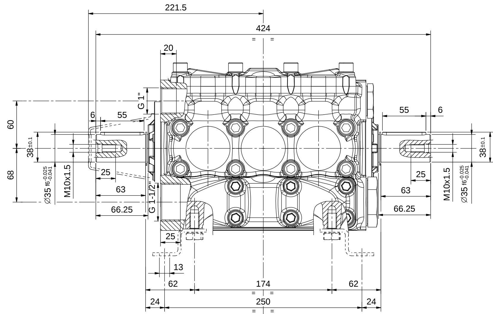
VERSIONE DOPPIA PRESA DI FORZA DIAM.35
