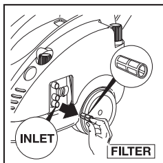
Den Filter aus dem Wassereinlaufstutzen herausziehen.
